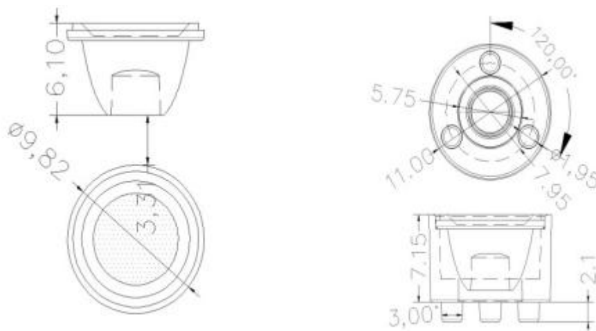
透镜外形尺寸 Len profile dimensions
