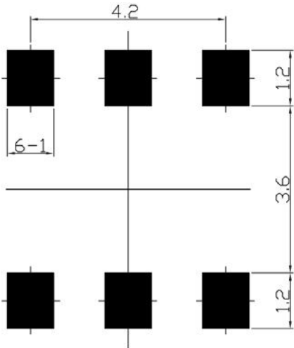
推荐焊盘尺寸图
