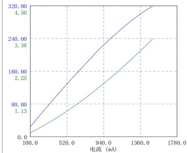
红外辐射强度 (mW/sr) 功率 (W)
